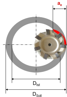
innen zirkular Fräsen
