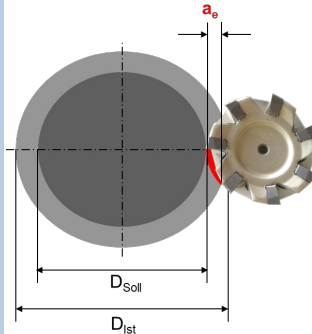
außen zirkular Fräsen
